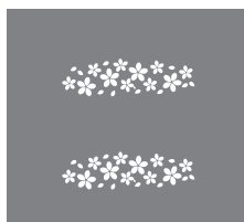
ヘアバンド
